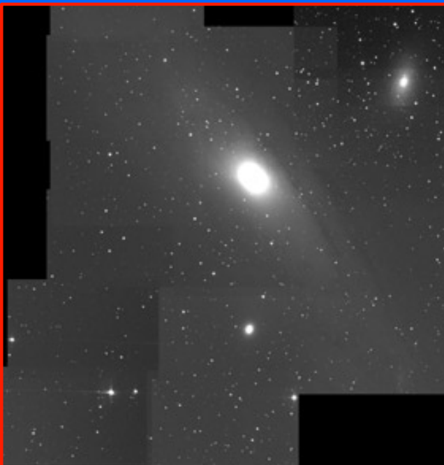
Messier 31 (décembre 2005)
