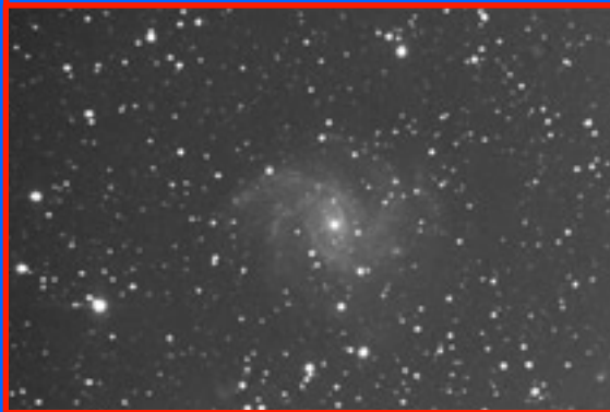
NGC 6946 (janvier 2006)
