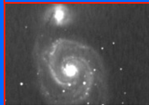
Messier 51 (janvier 2006)
